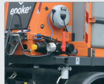
2" oder 3" Anschlusskupplung zur Befüllung/Entleerung
