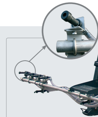
High-Speed Steuerung mittels Spratronic-Düsen. Steuerung bei allen Geschwindigkeiten bis auf zu 90 km/h möglich.
